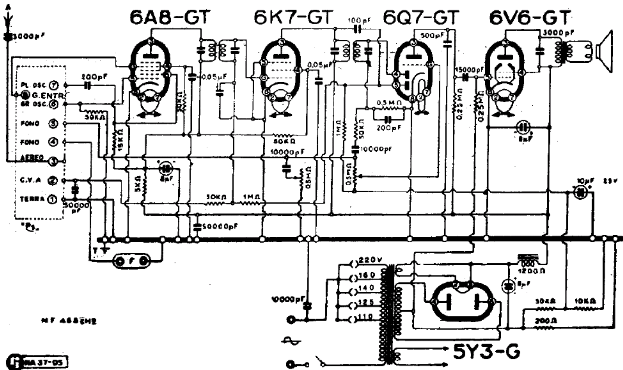
VARA RADIO - MOD. « 607 »
